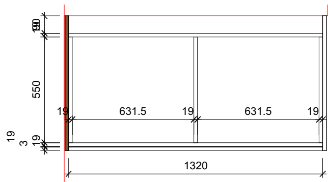
Sockelplan
